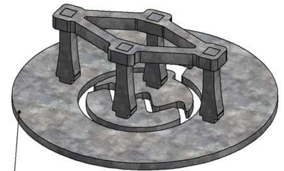
Steel Pottery Extruder Disk n° 108
